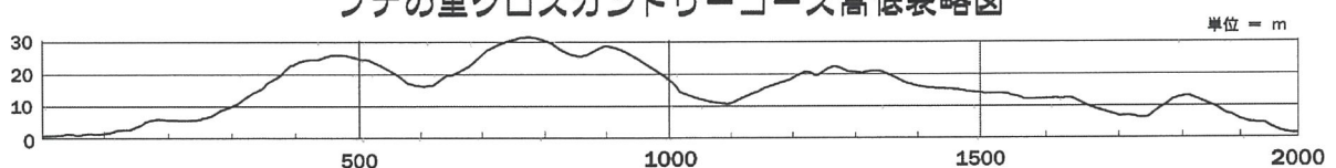
ブナの里クロスカントリーコース高低表略図
